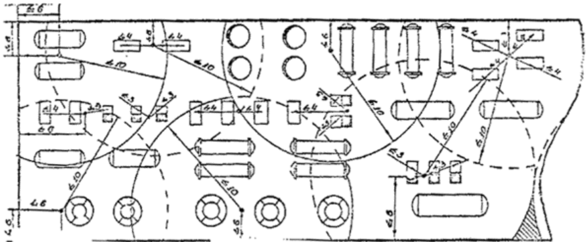
Примерный порядок расположения датчиков сигнализаторов до взрывных концентраций на открытой установке с наличием рассредоточенного расположения насосов:
