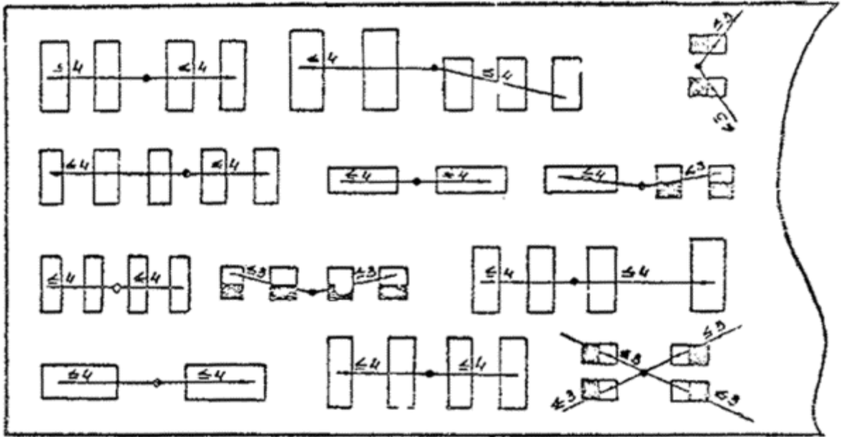
Примерный порядок расположения датчиков сигнализаторов до взрывных концентраций в насосных сжиженных газов и ЛВЖ:
